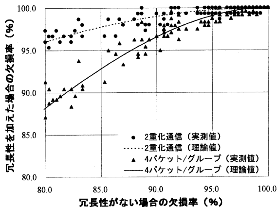
図 2: 冗長パケットの効果
