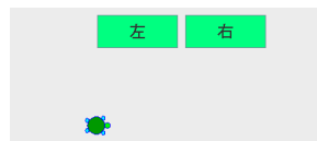
図 3.12: 左右ボタン
