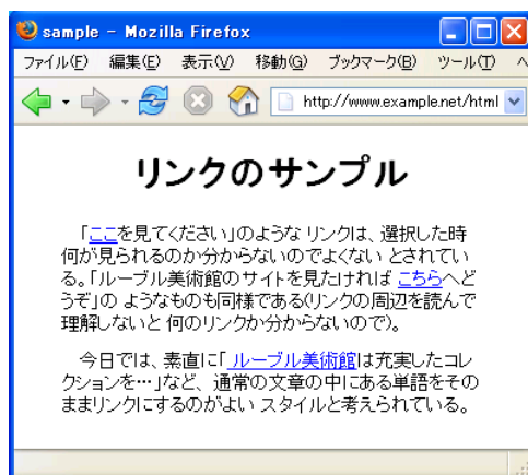
図 1.20: リンクの例
