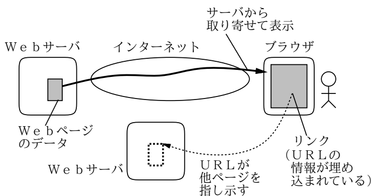
図 1.9: WWW の原理
